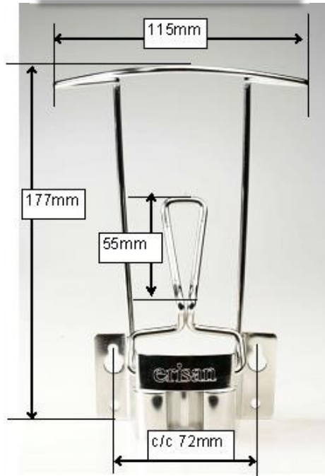
Dispenser-teline, lyhyt painike 8145
